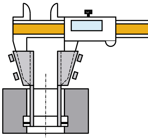
Nástavky na měření zápichů v hlubokých otvorech
