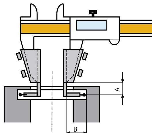
Nástavky na měření vnitřních zápichů (hodnoty A a B dle požadavků zákazníka)
