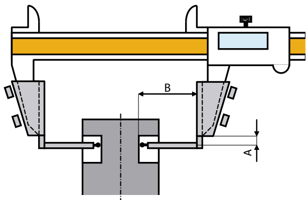
Nástavky na měření vnějších zápichů (hodnoty A a B dle požadavků zákazníka)
