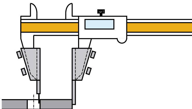
Nástavky k měření vzdálenosti otvoru od okraje (Ø drátků 4 mm, délka funkční části drátku 20 mm).
