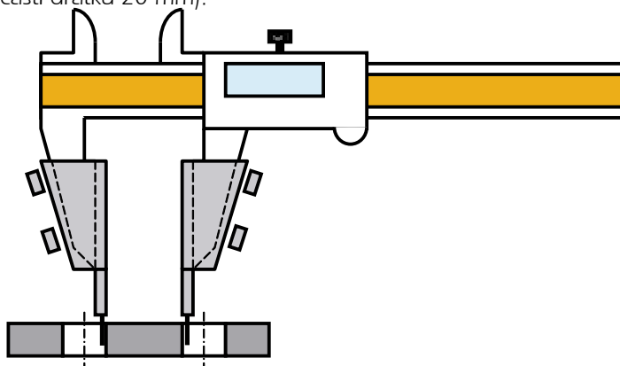
Nástavky k měření roztečí otvorů (Ø drátků 4 mm, délka funkční části drátků 20 mm).
