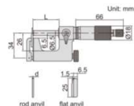
flat anvil
