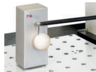
Kalibrační etalon s dvěma kuličkami
