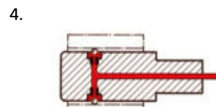
4. Měření průměrů průchozích otvorů s hlavici s kuličkovými kontakty
