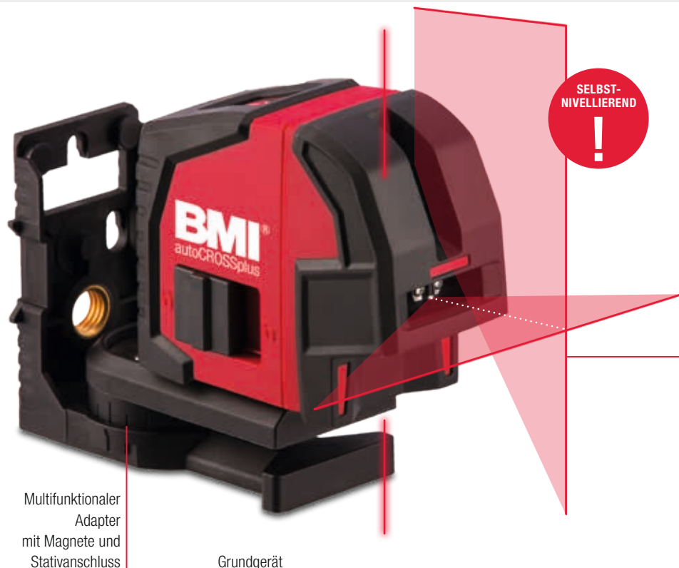
Grundgerät
